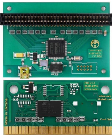
Figura 4.41: Programador i PCB de Krikzz
