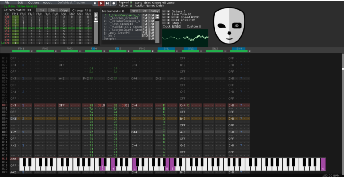
Figura 4.28: Interfície Deflemask
