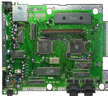
Figura 2.2: Placa base Mega Drive model europeu
