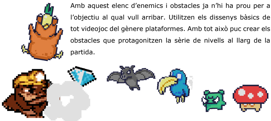
Figura 4.23: Elenc d'enemics
